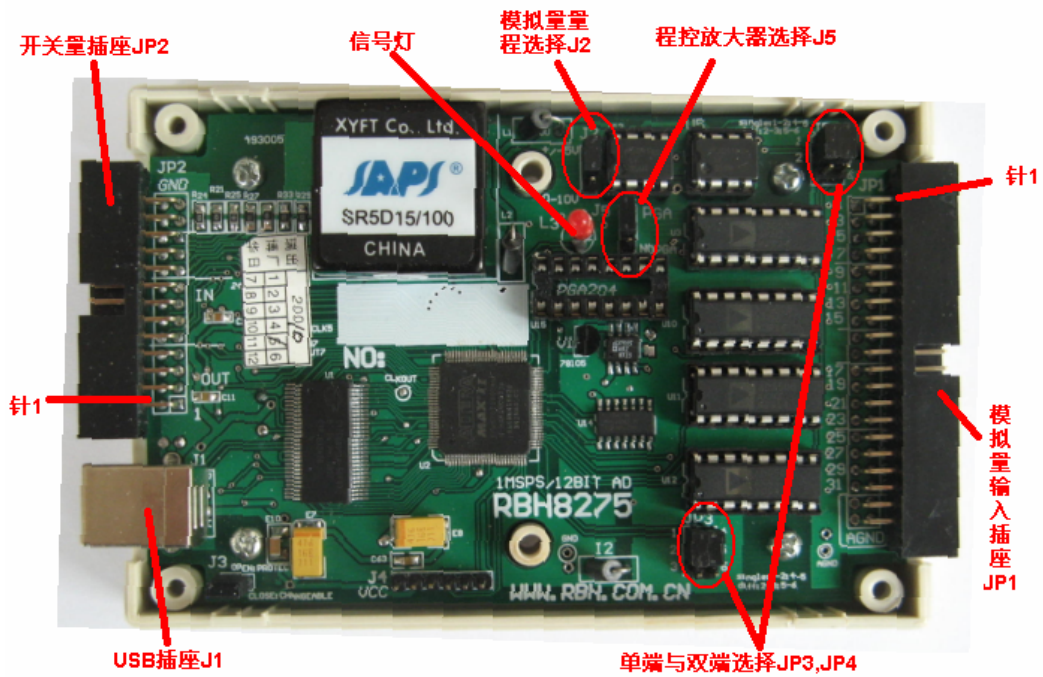
图 2 RBH8275 的电路板
