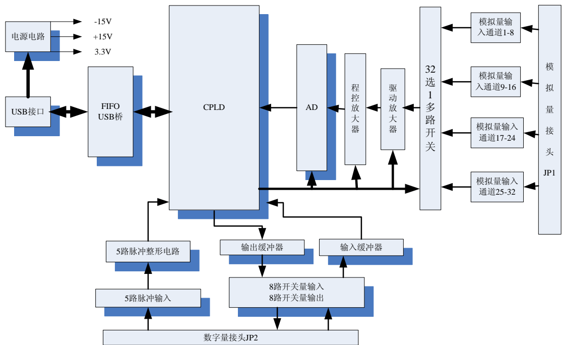
图 1 原理框图
