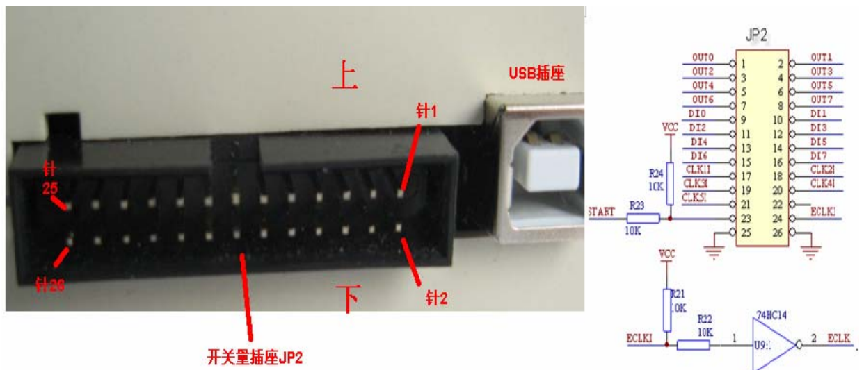
图 4 数字量接头 JP2 的定义
