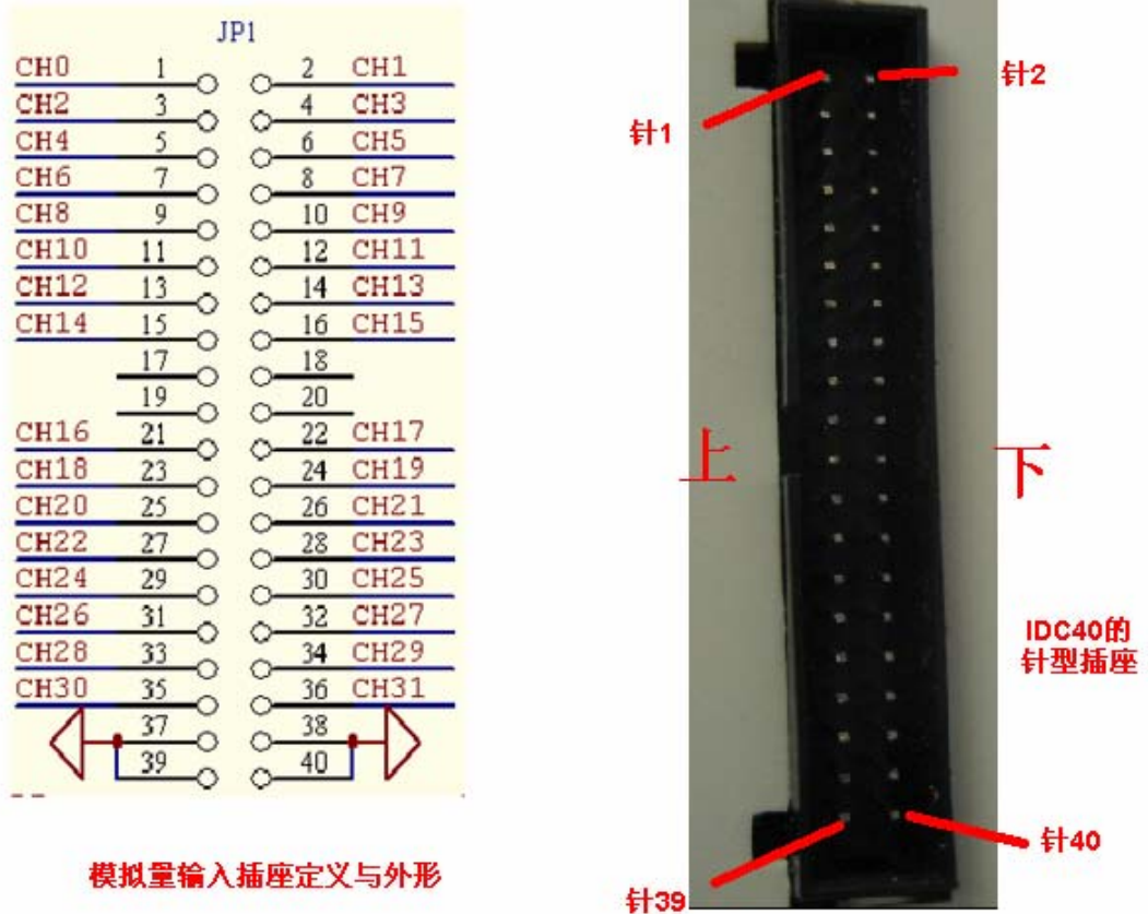
图 5 模拟量输入插座 JP1 的定义及外形
