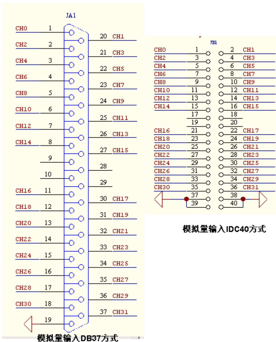
图 5 模拟量通道
