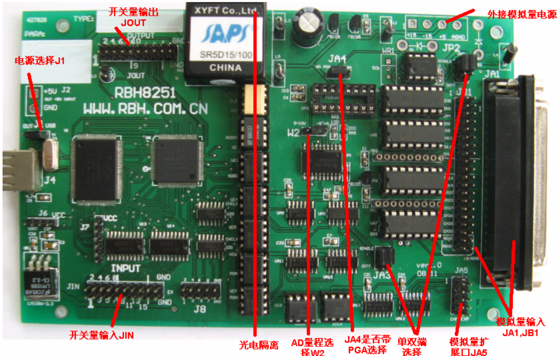
图 2 实物及接头定义
