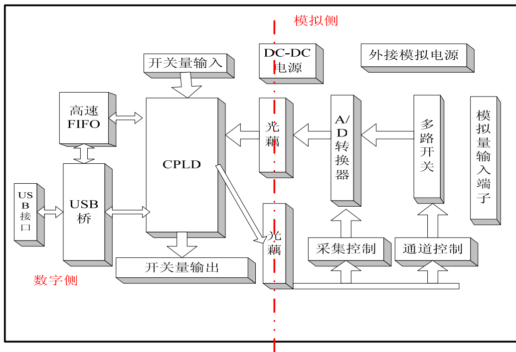
图 1 原理框图
