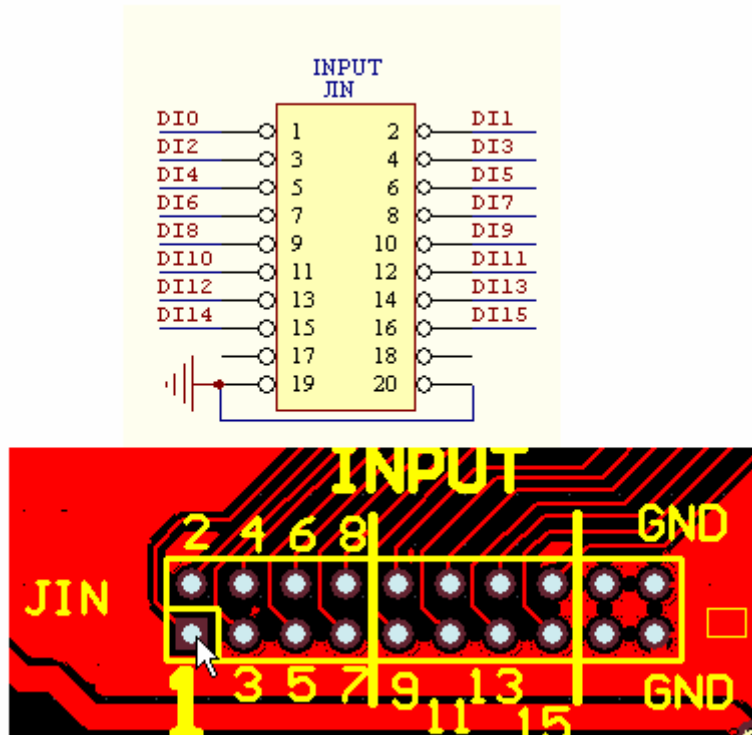
图 3 开关量输入的原理与接线图
