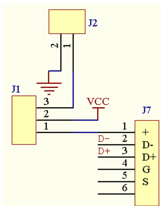
图 6 数字电源的接线原理
