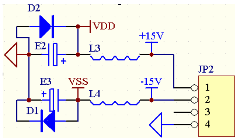
图 7 模拟电源的接线原理
