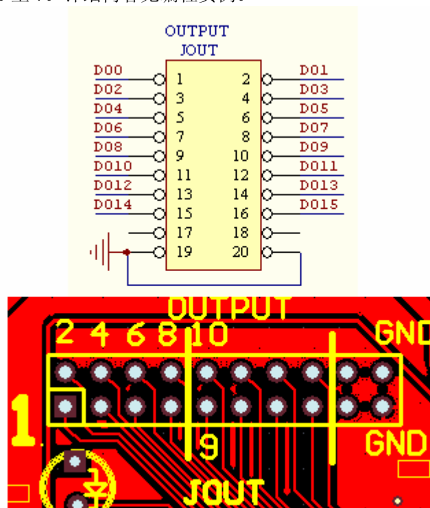
图 4 开关量输出的原理与接线图
